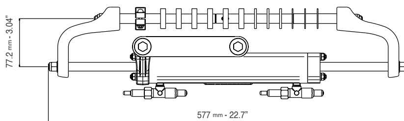
UC81-OBF DIMENSIONS
