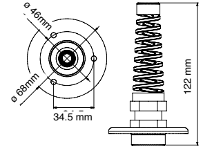
R5 DIMENSIONS
