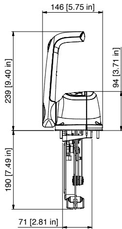
B501 - B502 Dimensions
