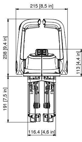
B502CHT/L - B502BT/L Dimensions
